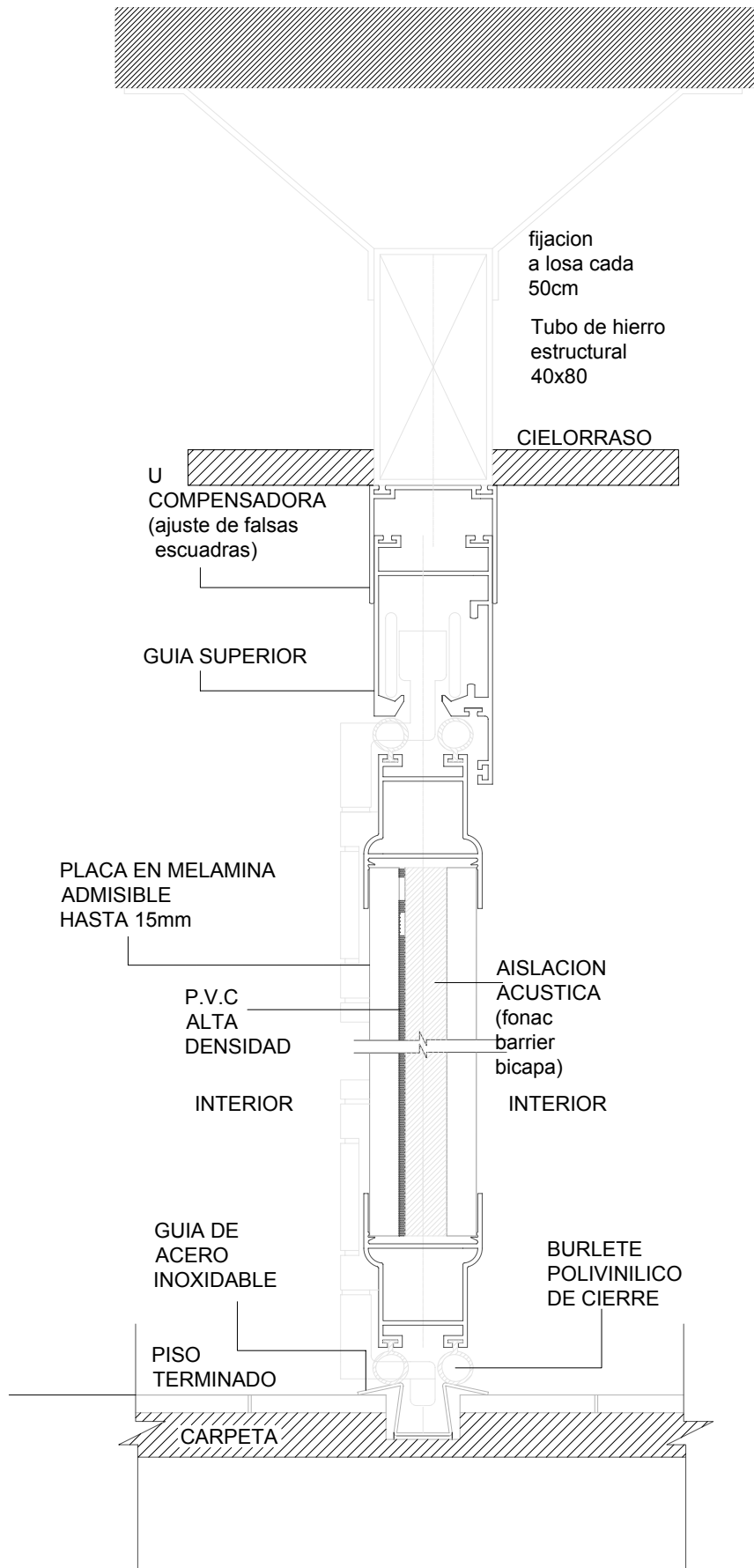
DETALLE: DIVISOR PLEGABLE CON PANEL COMPUESTO 38MM
