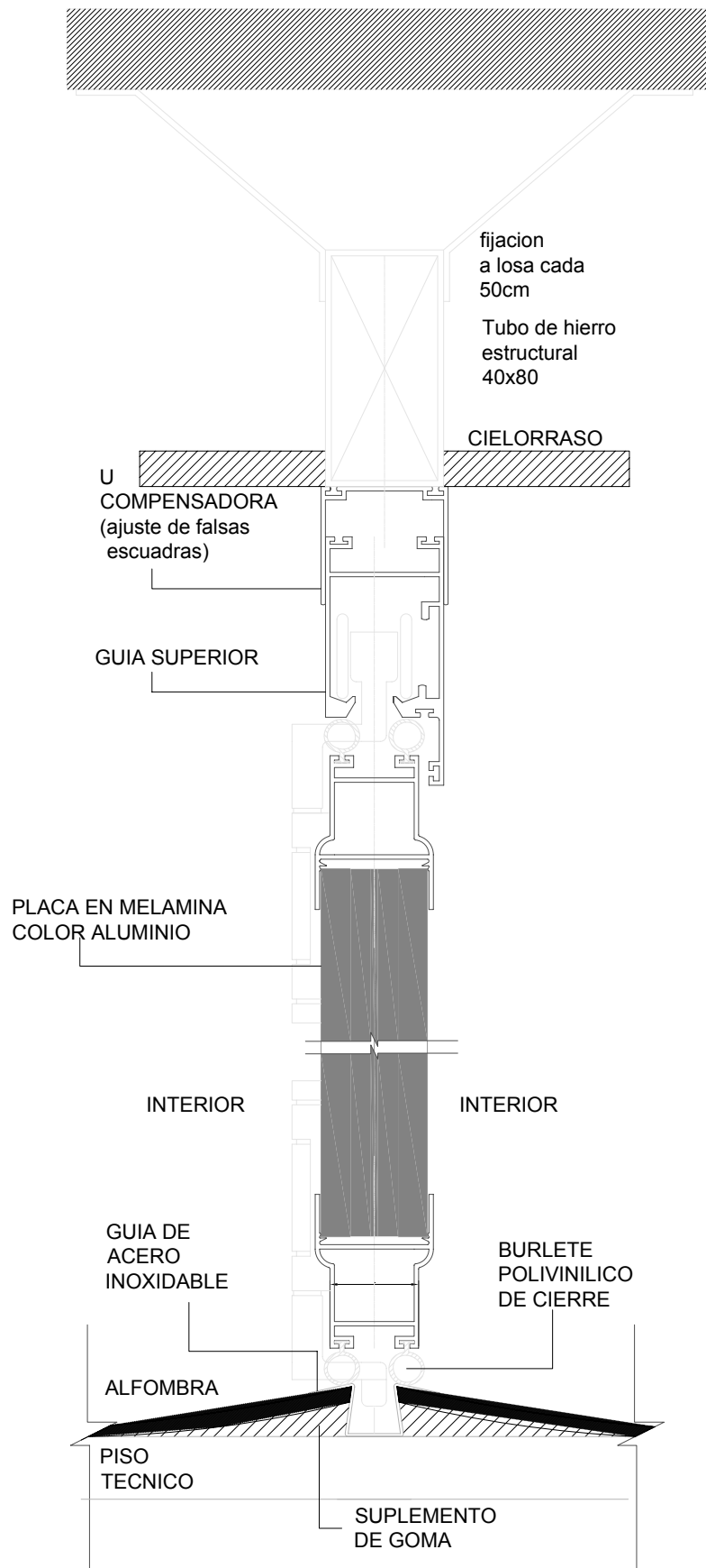
DETALLE: DIVISOR PLEGABLE PANEL COMPUESTO 38MM
